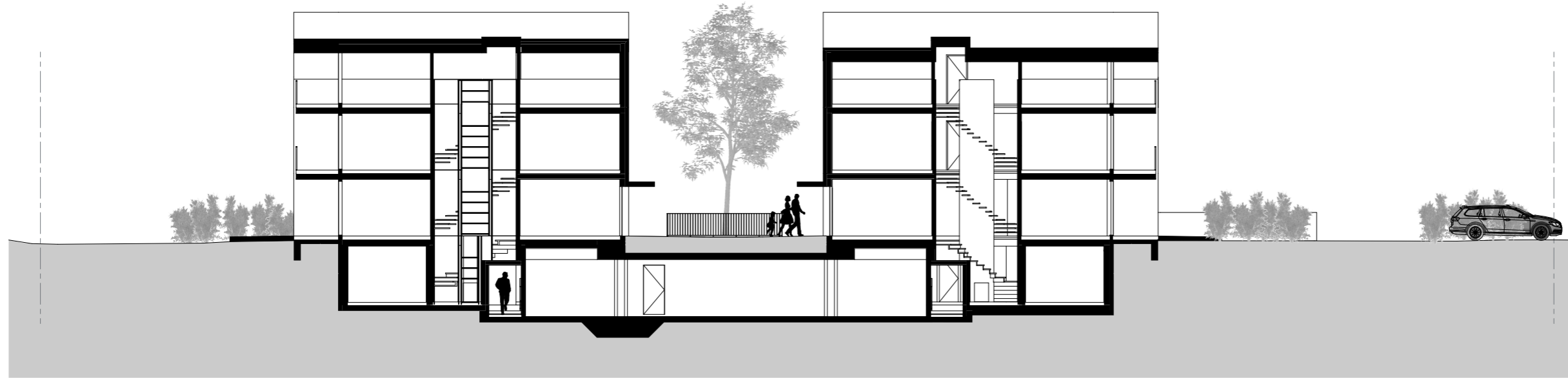
Schnitt S02
