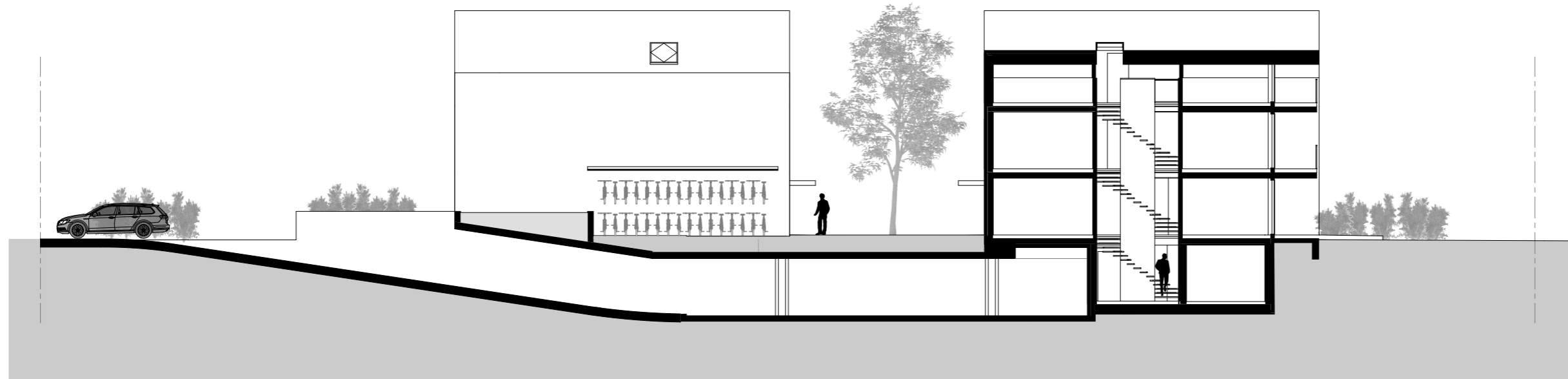
Schnitt S03
